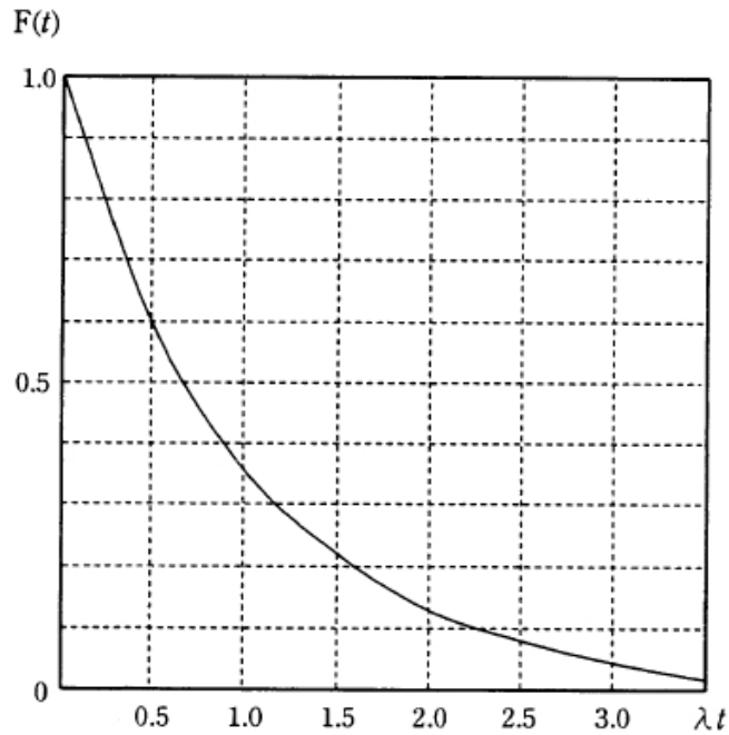
指数関数 F(t) = \exp(-\lambda t)
