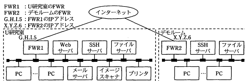
図 ネットワーク構成
