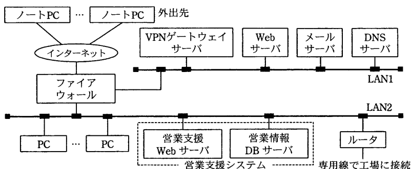
図1 W社本社ビルの情報システムの構成
