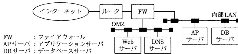
図 Xシステムのネットワーク構成
