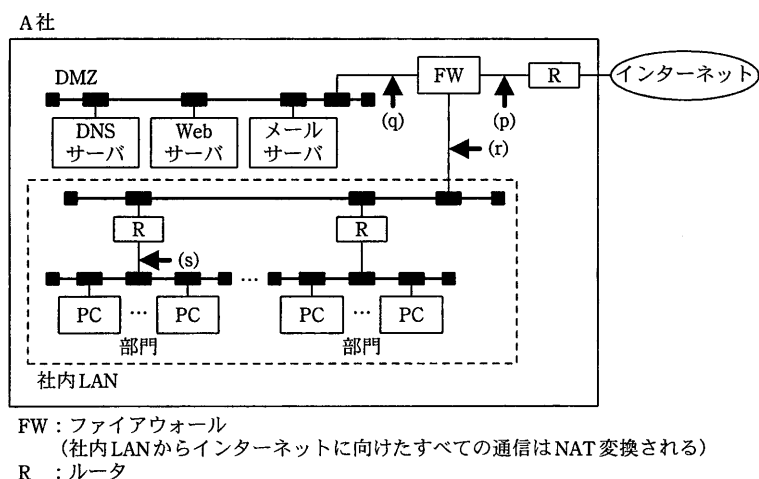
図1 A社の業務用ネットワークの構成
