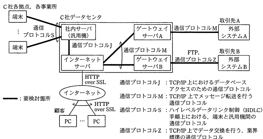
図2 Yシステムにおいて通信データの保護を検討すべき箇所
