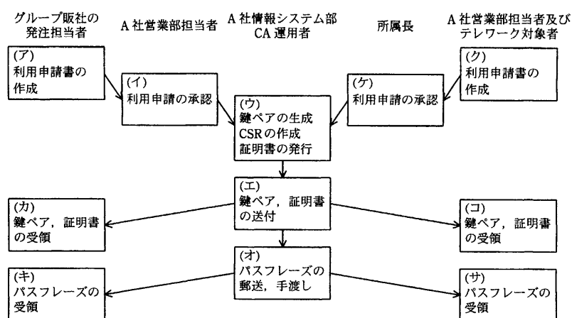
図1 証明書発行の運用フロー
