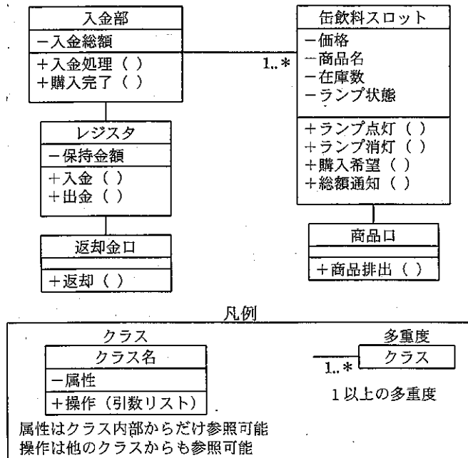
図1 最初のクラス図
