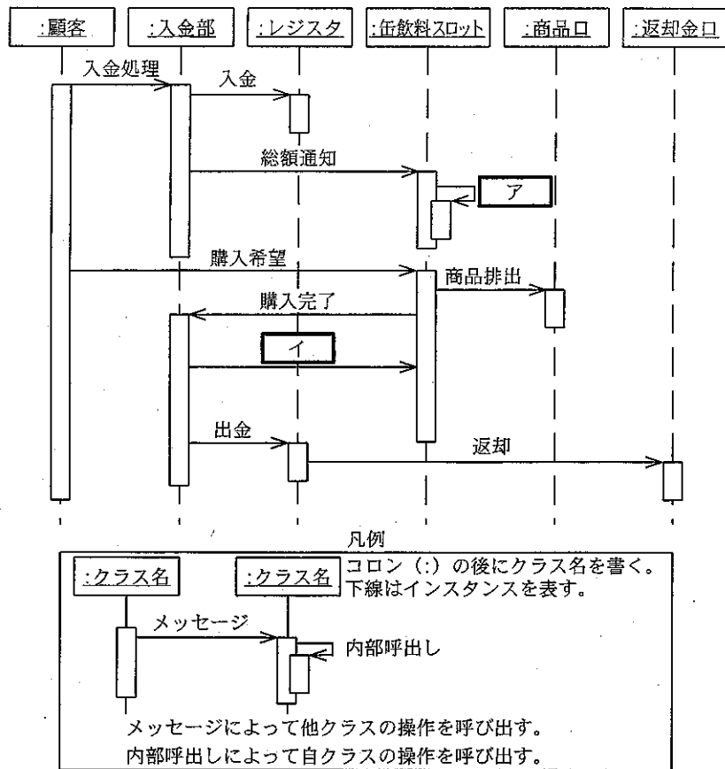
図2 最初のシーケンス図
