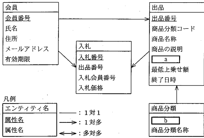
図2 E-R図
