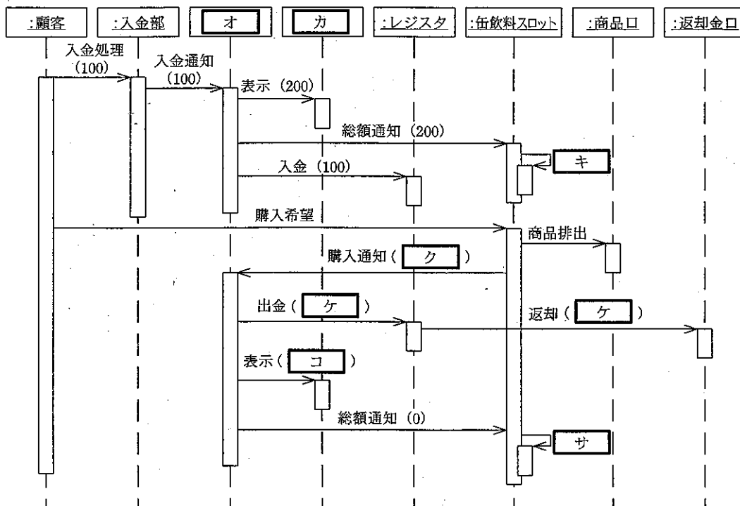
図4 修正したシーケンス図
