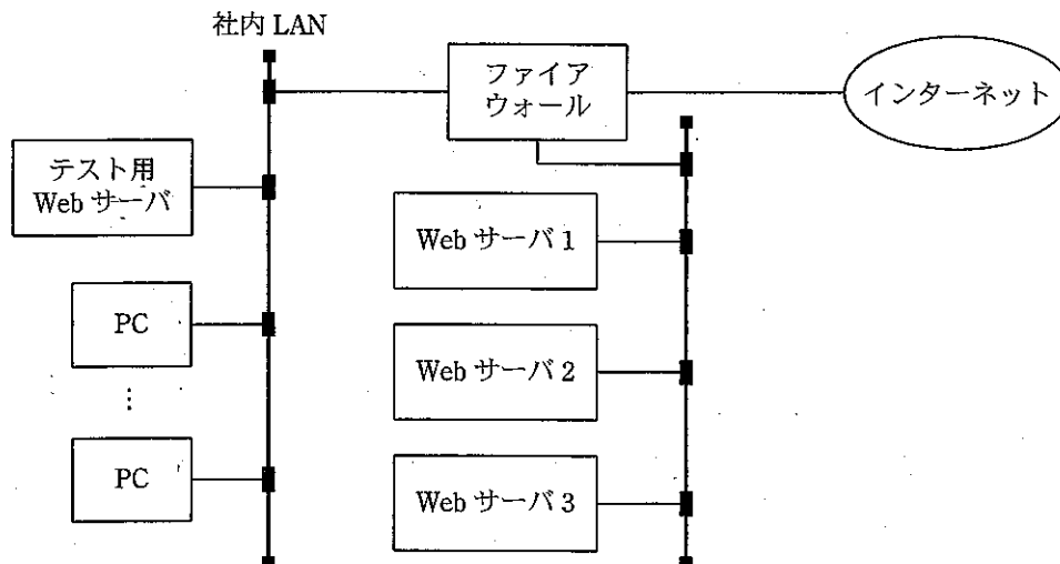
図1 A社の情報提供システムの構成
