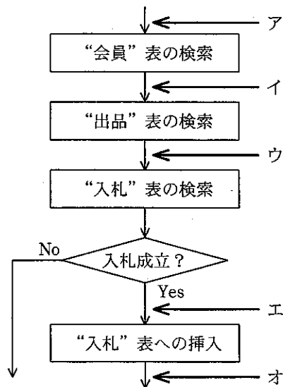
図 3 入札操作の処理
