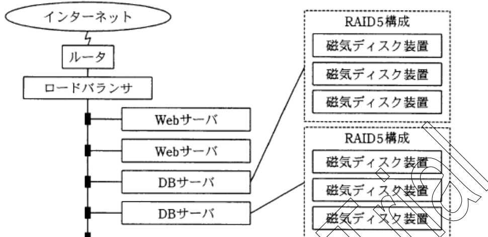
図 2 新システム構成
