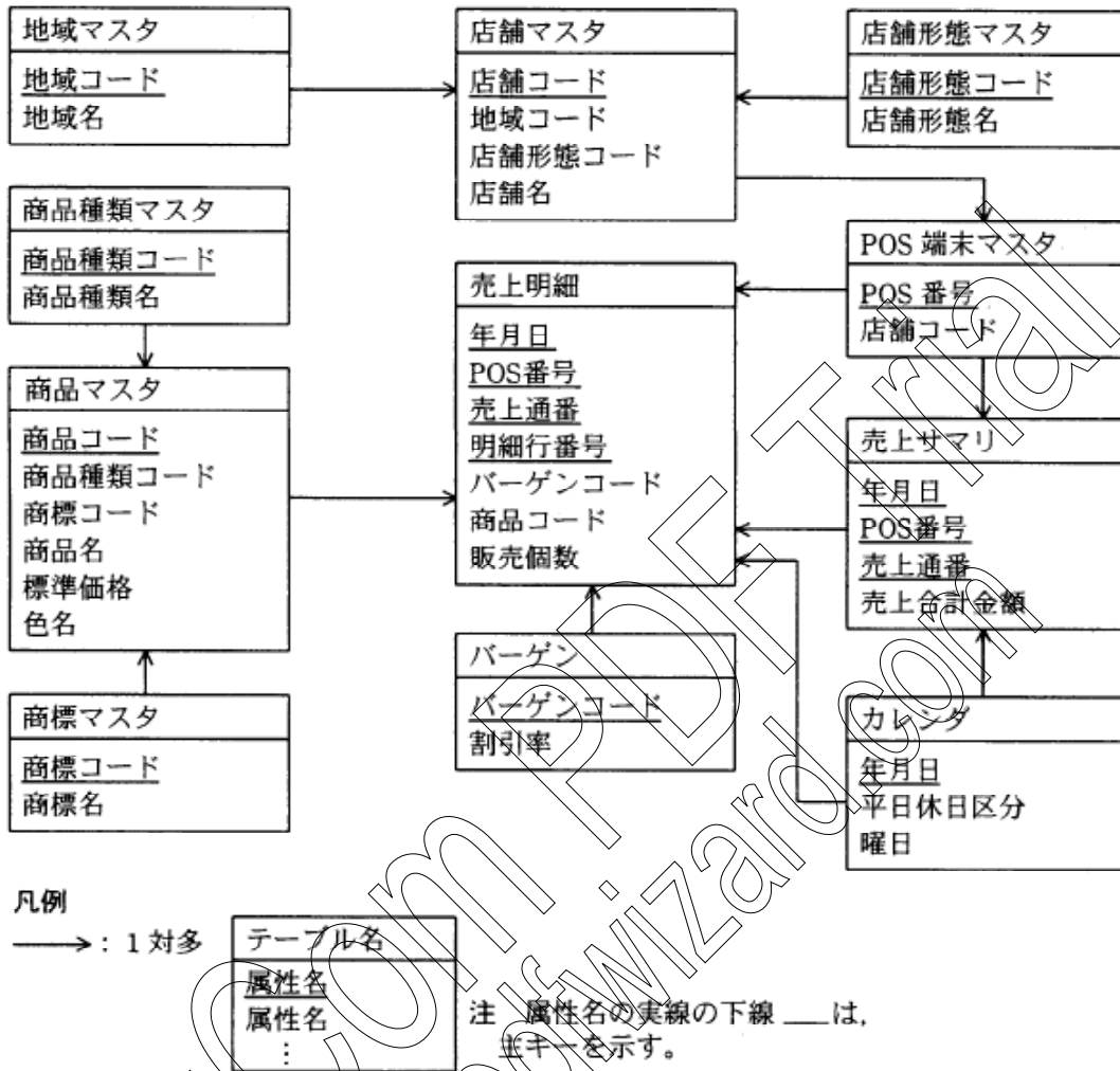
図 1 販売システムの E-R 図
